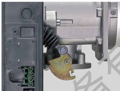
RS 34-44/M MZ 系列燃烧器可变线凸轮示例。
