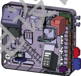
RS 34-44/M MZ 型燃烧器电气部件外壳及电气连接用“插头-插座系统”示例。
