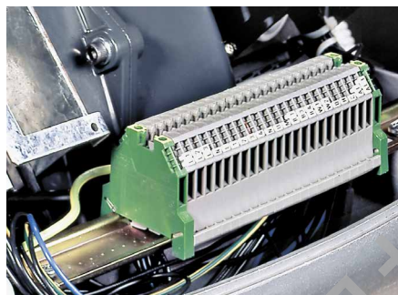
RS 70-100-130-190-250/M 型燃烧器电气连接用接线端子板示例。
