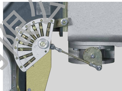
RS 250/M MZ 系列燃烧器可变线凸轮示例。
