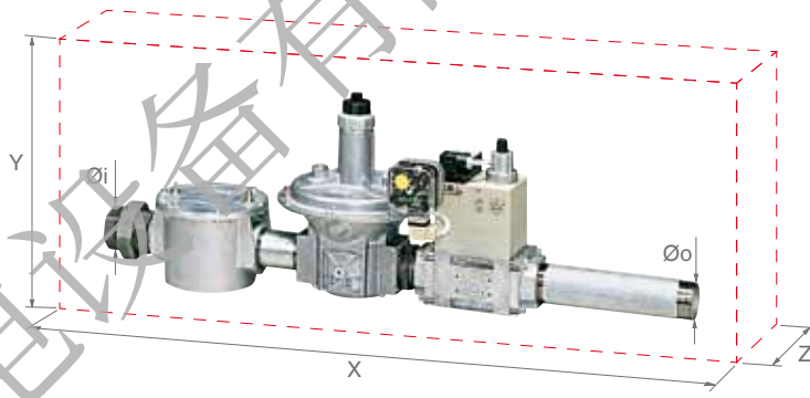
无泄漏检测仪的“组合式”燃气阀组示例
